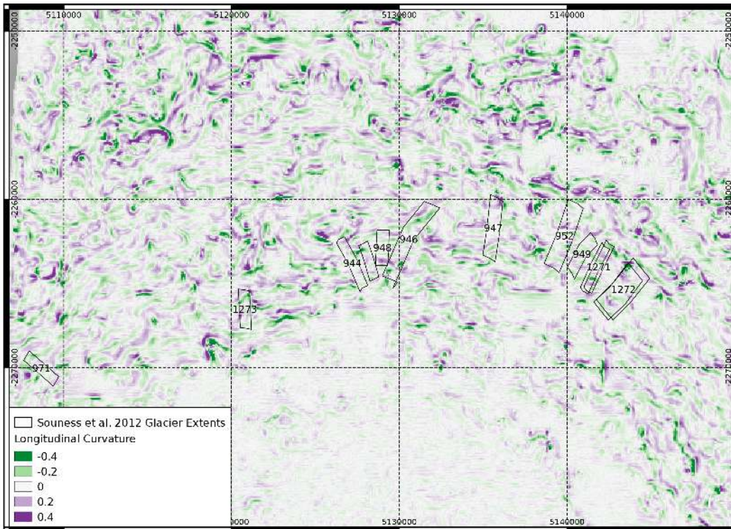
(a) Longitudinal Curvature
